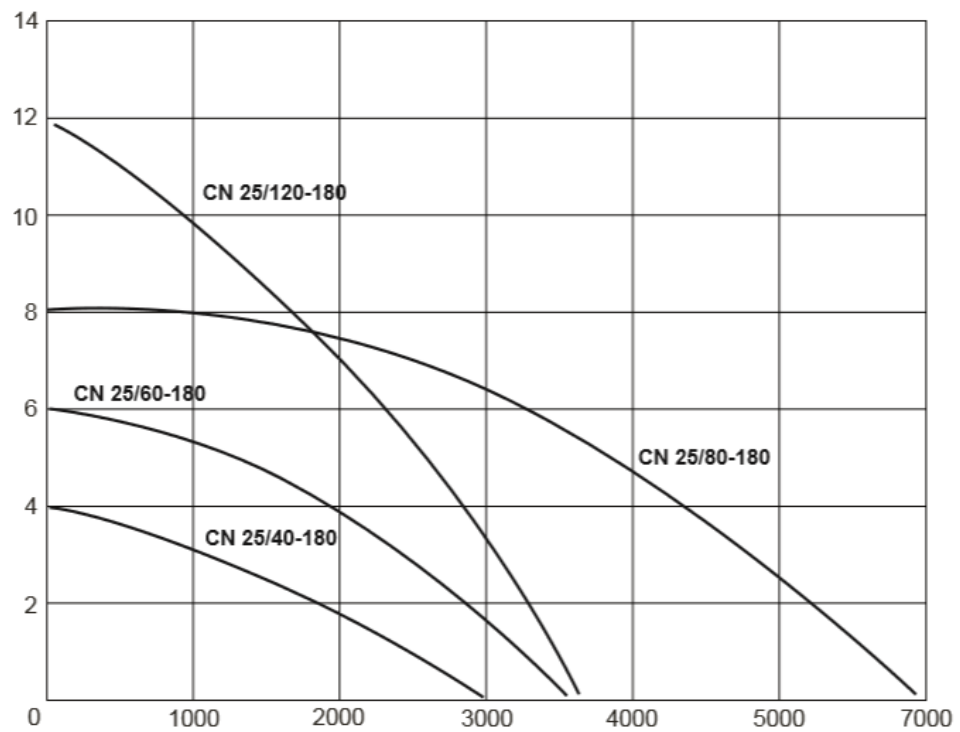
Графики производительности циркуляционных насосов WWQ серии CN
